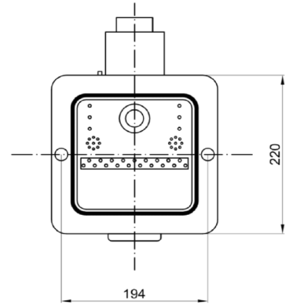
Abmessungen der Befestigungslöcher
