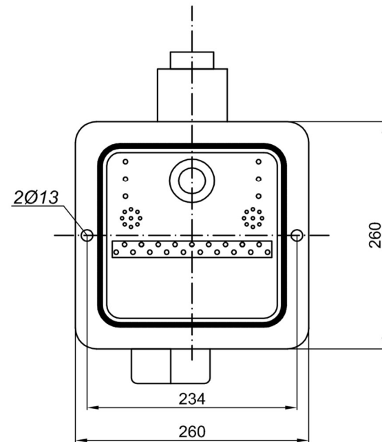
Abmessungen der Befestigungslöcher
