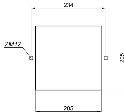
Abmessungen der Befestigungslöcher
